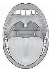
Стадия I (>25% <50%)
