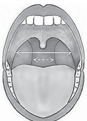
Стадия II (>50% <75%)
