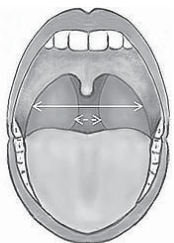
Стадия III (>75%)
