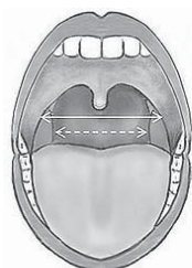
Стадия 0 (<25%)
